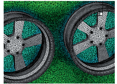
Verchromung von Autorädern: Gitter für die numerische Simulation (Elyca)
