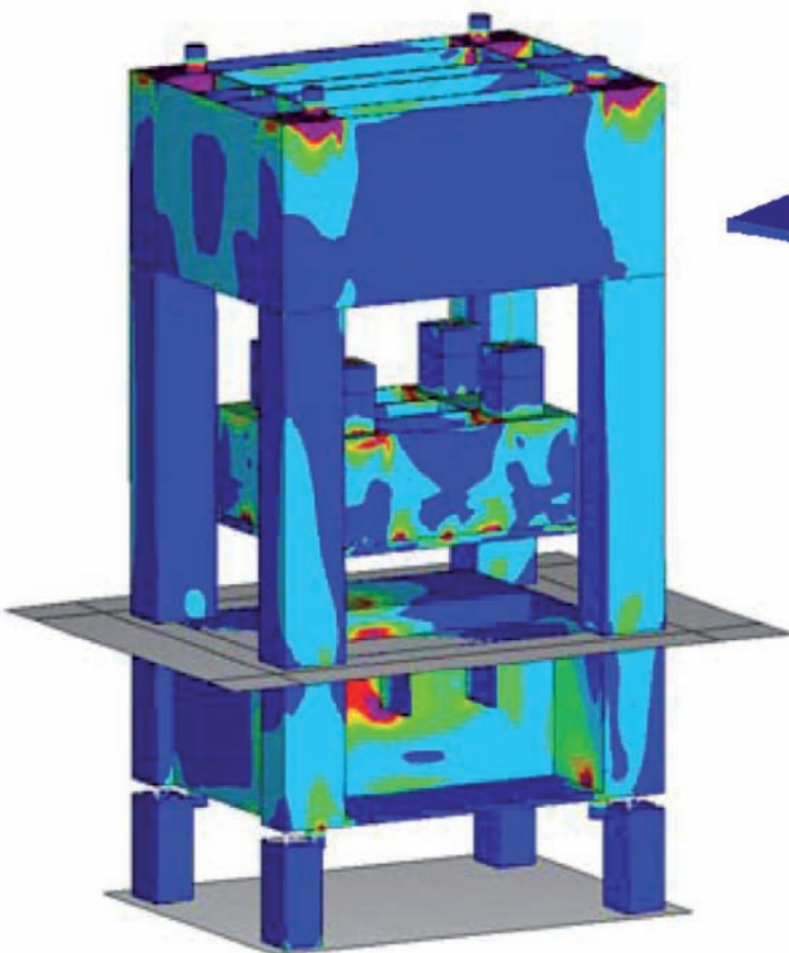
Gekoppelte Simulation elastischer Umformwerkzeuge.
