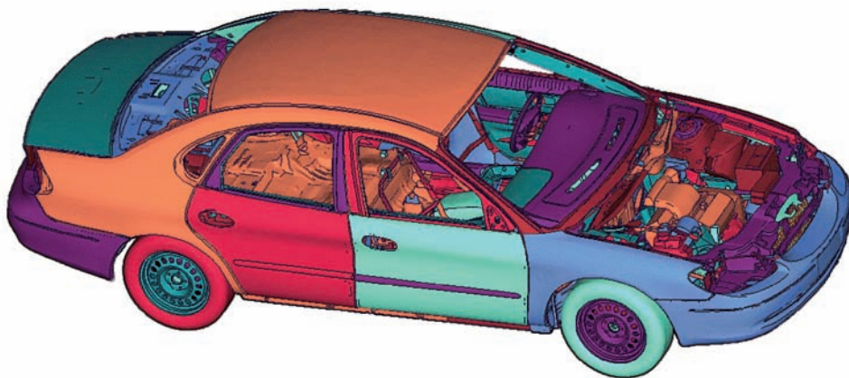
Finite-Elemente-Modell eines Ford Taurus für die Crash-Simulation mit etwa einer Million Gitterpunkten. Das Modell stammt vom National Crash Analysis Center (NCAC), Ashburn Virginia, USA.
