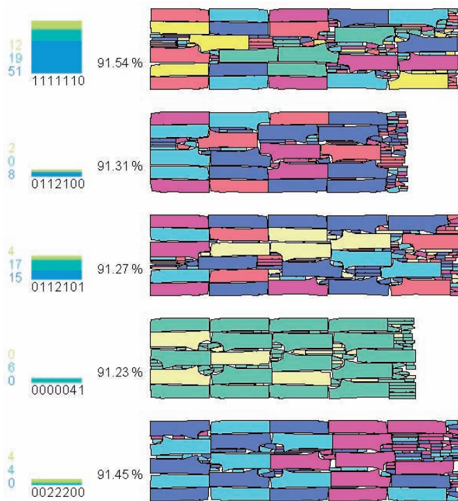
Produktionsplan für eine Hose in sieben Konfektionsgrößen und drei Stoffen mit berechneten Materialkosten.
