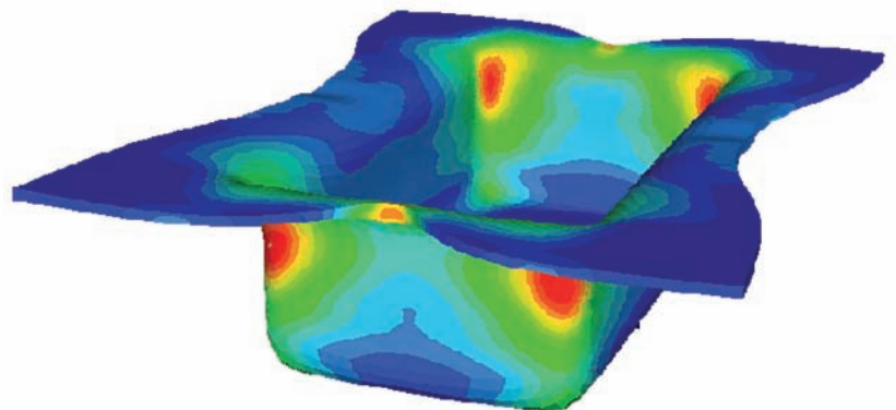
Gekoppelte Simulation elastischer Umformwerkzeuge.
