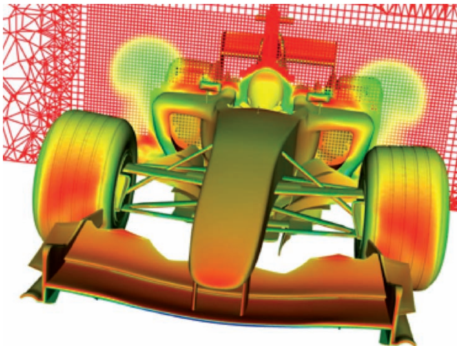
Vernetzung des Modells eines Rennwagens der Formel 1: Die Bild zeigt eine einzelne Gitterschicht. Das gesamte Gitter besteht aus etwa 100 Millionen Zellen und ist in Oberflächennähe extrem fein (siehe rechts).
