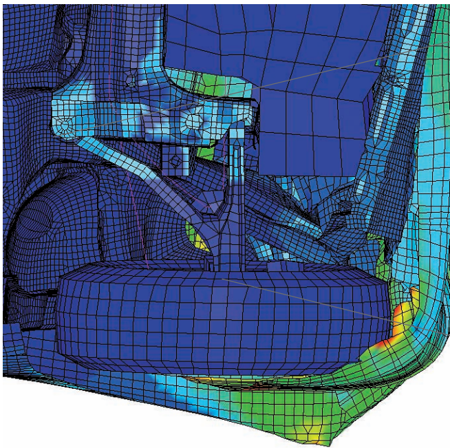
Bild 2: Streuung von Knotenpositionen in unterschiedlichen Simulationsläufen.
