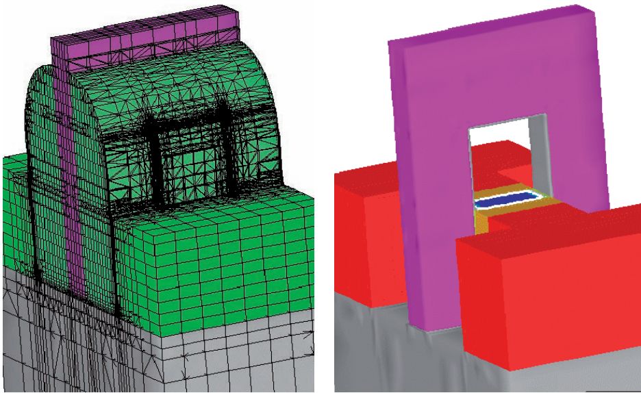
Device-Simulation: Gitter und Dopingprofil eines FinFET-Transistors (Synopsys Inc.)
