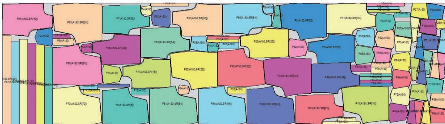
Verschachtelung von Polstermöbelteilen auf Lederhäuten. Die Farben repräsentieren unterschiedliche Qualitäten auf der Lederhaut und unterschiedliche Qualitätsanforderungen auf den Teilen.
