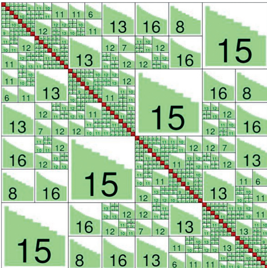
Bild 3: Typische hierarchische Blockstruktur einer H-Matrix. Jeder grün eingefärbte Block ist im speicherreduzierten Format dargestellt, wobei die Nummern dem Grad der Reduzierung entsprechen.
