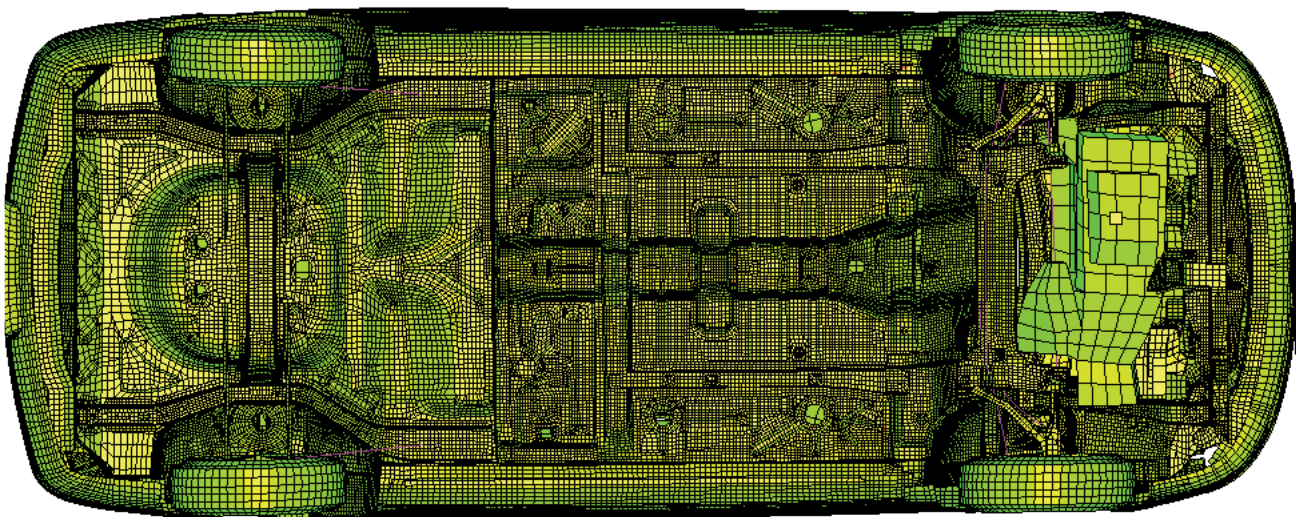
Bild 1: Ein Crash-Szenario für das Modell Neon von Chrysler.
