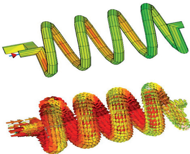
Bild 1: Oberflächenstrom und Feldbild einer Helix-Antenne
