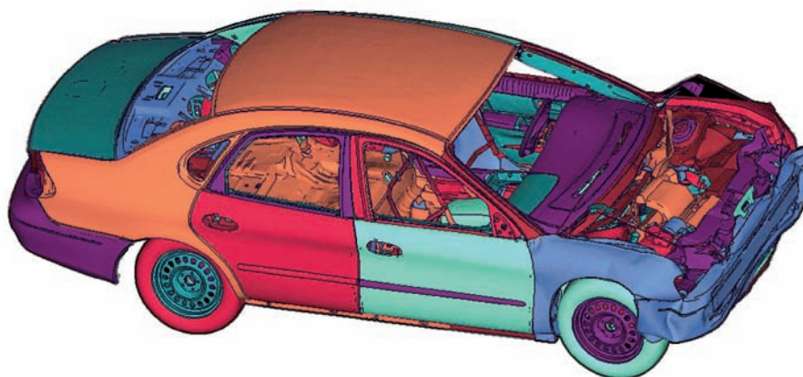
Simulationsergebnis eines Frontcrash mit vollständiger Überdeckung zwischen Modell und Barriere.
