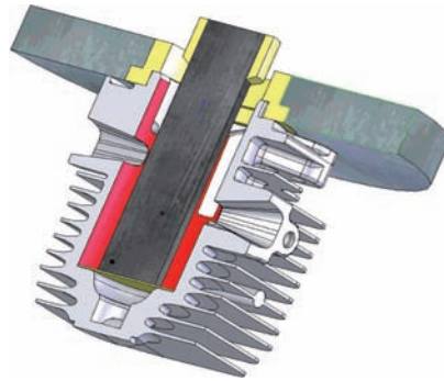
Geometrie zur Verchromung eines Verbrennungszylinders (Elyca)
