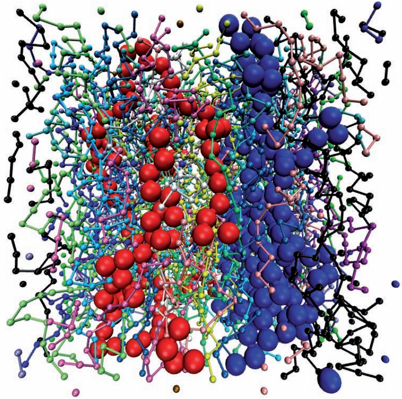
Modell einer Polymerschmelze, zwei Polymere (rot und blau) sind hervorgehoben.
