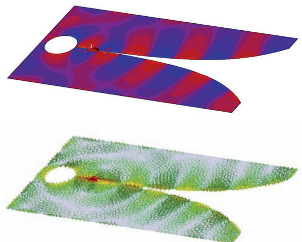
Bild 2: Oberflächenstrom und Feldbild einer Vivaldi-Antenne
