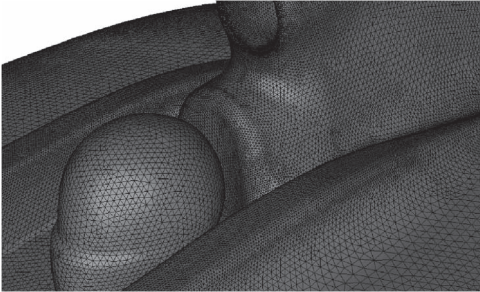
Oberflächengitter in der Umgebung des Fahrers (Bilder mit Dank an Sauber-Petronas und Fluent)
